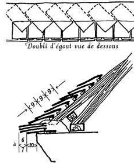
La bordure à l'égout doit dépasser la corniche et écarter ainsi l'humidité
