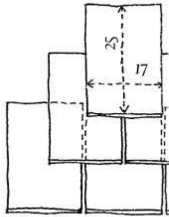
Assemblage des 3 recouvrement.
